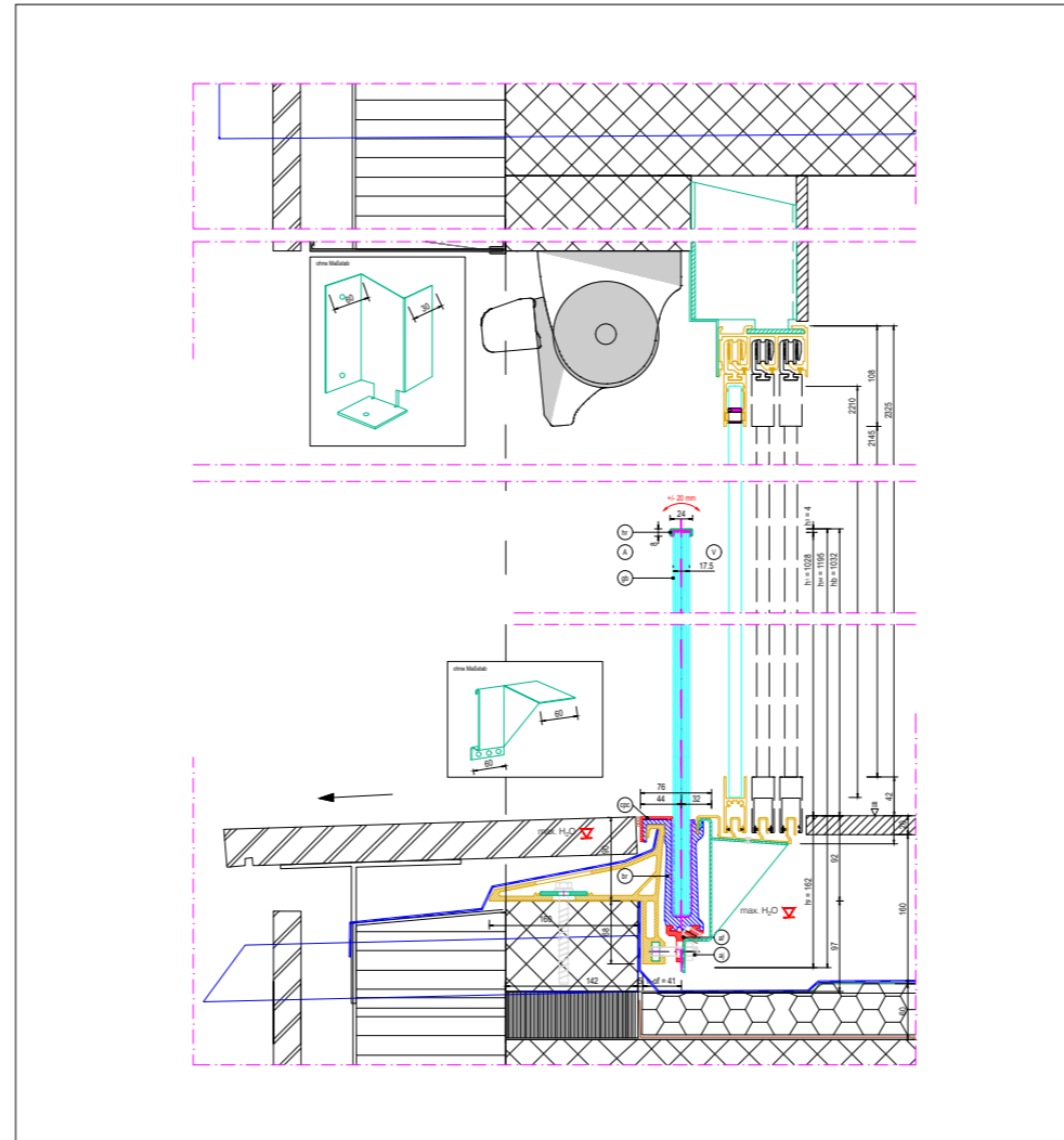
Deckenhohe Lösung als Kombination aus GM RAILING® UNI PART und GM TOPROLL® 10/14
