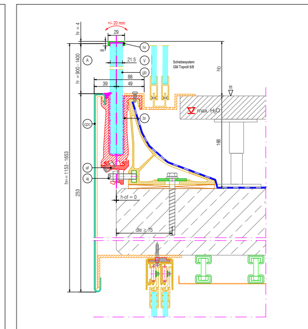
Raumhohes Kombisystem
