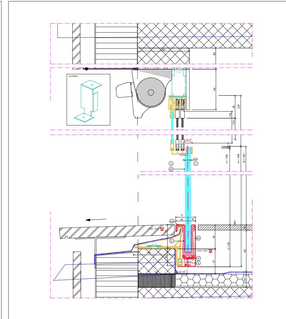
Schiebesystem GM TOPROLL® 6/8 aufgesetzt auf das Glasgeländer-System GM RAILING® UNI PART
